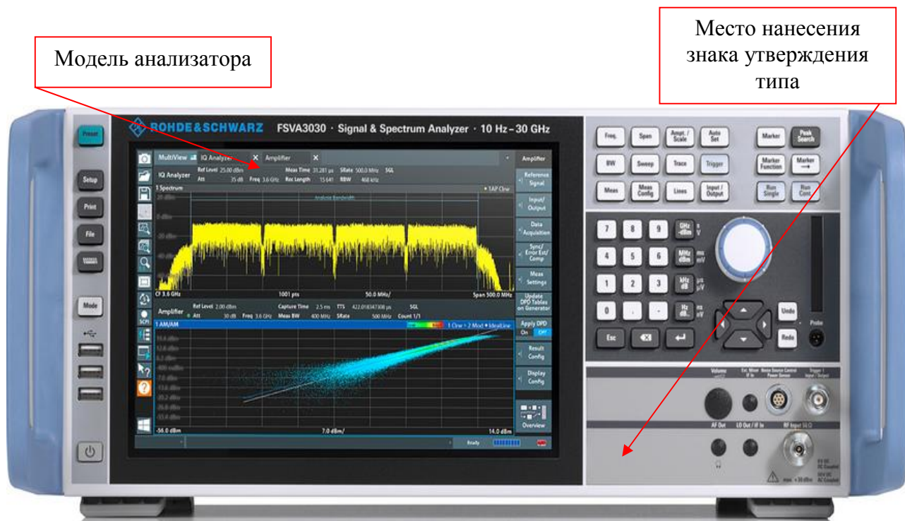
Рисунок 1 - Общий вид анализаторов спектра FSV3004, FSVA3004, FSV3007, FSVA3007, FSV3013, FSVA3013, FSV3030, FSVA3030, FSV3044, FSVA3044
